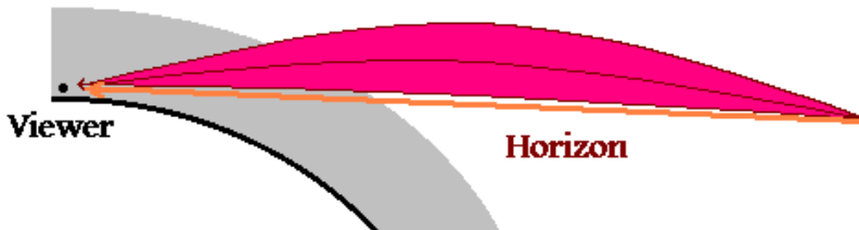
Figure 2: courbure lumière rouge horizon
