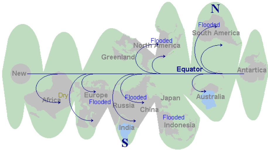
Figure 4: circulation des vents après PS2
